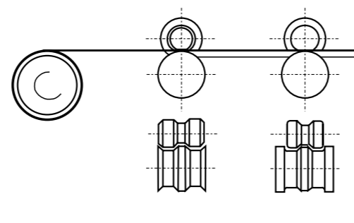
tussenstappen bij een rolvormer
