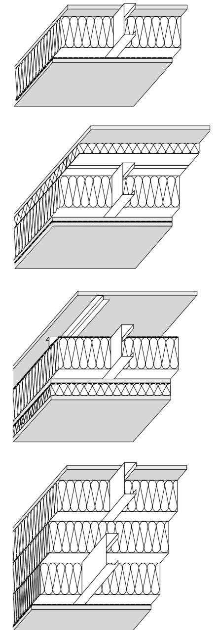
74. Verschillende opbouwen van staalframebouw wanden.
