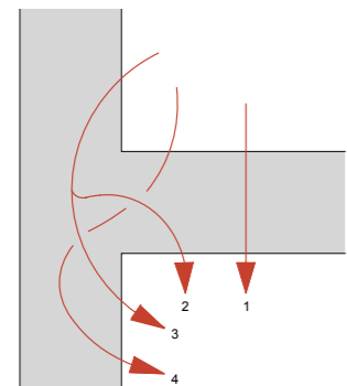
59b. Gecombineerde overdrachtswegen (4x) door het scheidende en het flankerende bouwdeel.
