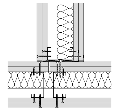
62. Akoestisch 'goed' gedetailleerde wandaansluiting met gesloten voeg en een scheiding in de doorgaande bekleding.
