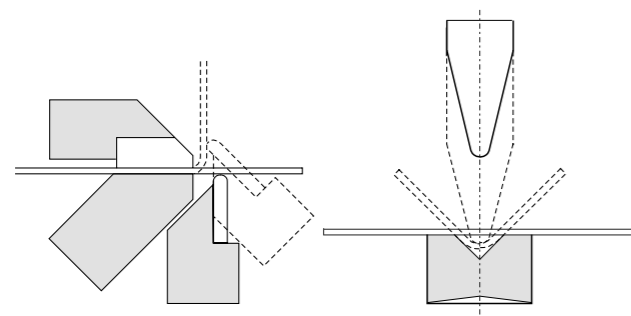
zetbank met 'zij-pers'
