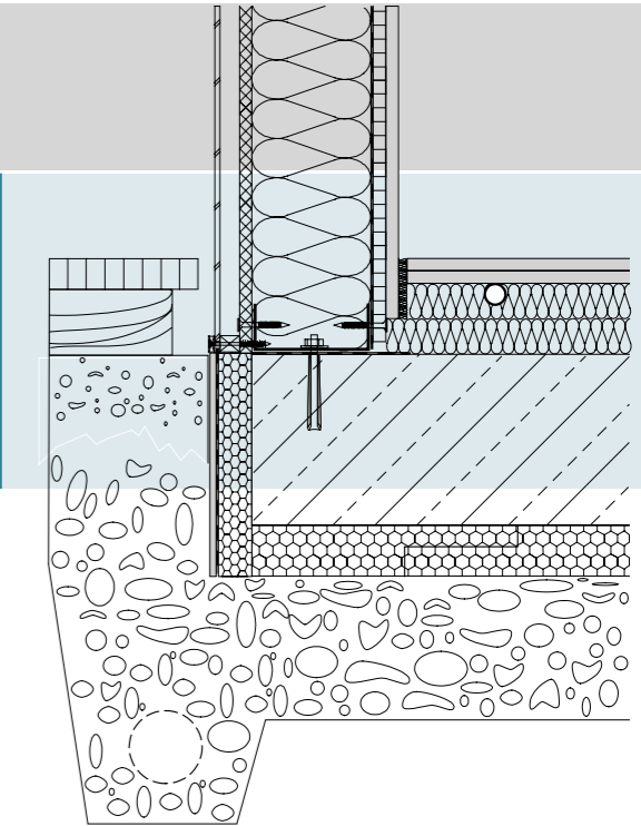
29. Aansluitdetail van een staalframebouw wand op een niet-onderheide fundering.
