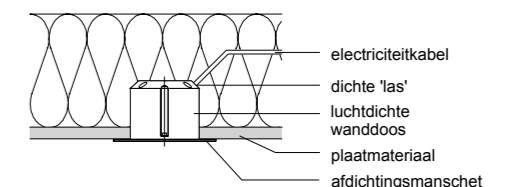
89. Een luchtdichte uitvoering van een wandcontactdoos.
