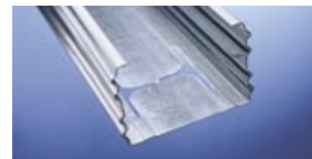
53b. Akoestisch metal-studprofiel met rillen in de flenzen.
