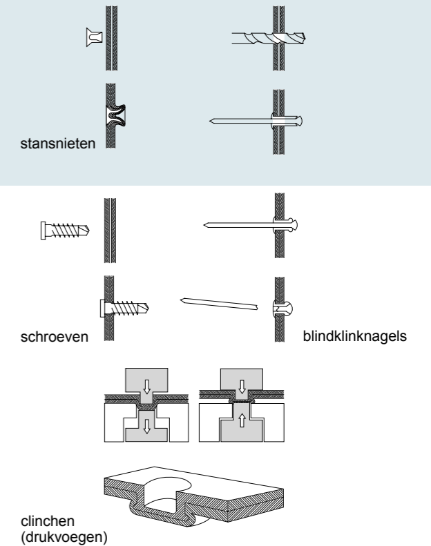
44. Verbindingsmogelijkheden tussen koudgevormde profielen onderling.
