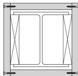
110. Brandwerende gipsbekledingen voor staalprofielen.
