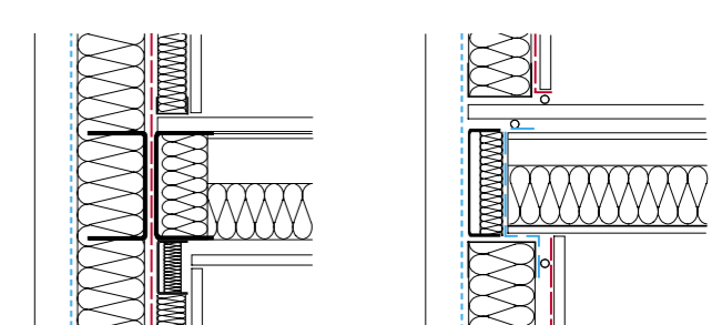
93. Verschillende aansluitingen van vloeren op buitenwand voor de balloon- en platformmethode met lucht- en winddichte uitvoeringen. De rode folie is dampremmend, de blauwe folie is dampdoorlatend.
