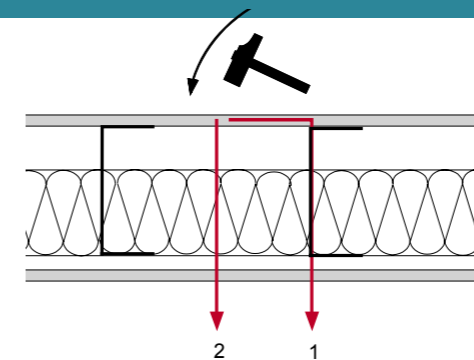
55. Contactgeluid bij staalframebouw vloeren 1. via de ligger; 2. via de holle ruimte.
