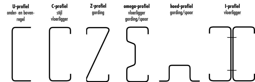
33. Doorsnedes van koudgevormde profielen voor de woningbouw.
