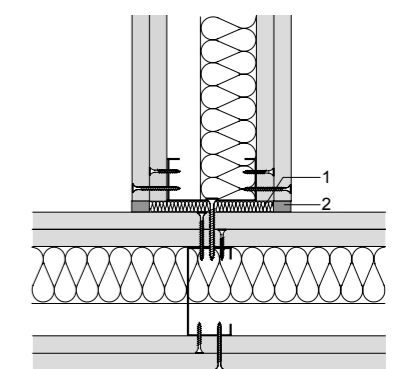
1 vulstroken van minerale wol 10 mm smeltpunt > 1000 °C 2 voegdichting
