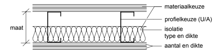
100. Mogelijkheden bij staalframebouw om de brandwerendheid te verbeteren.
