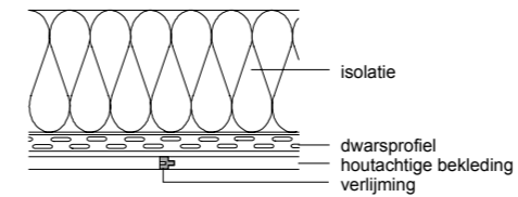
voegafdichting door verlijming
