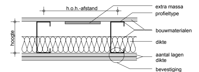
49. Akoestische parameters bij een aan weerszijden bekleed staalframebouw element.
