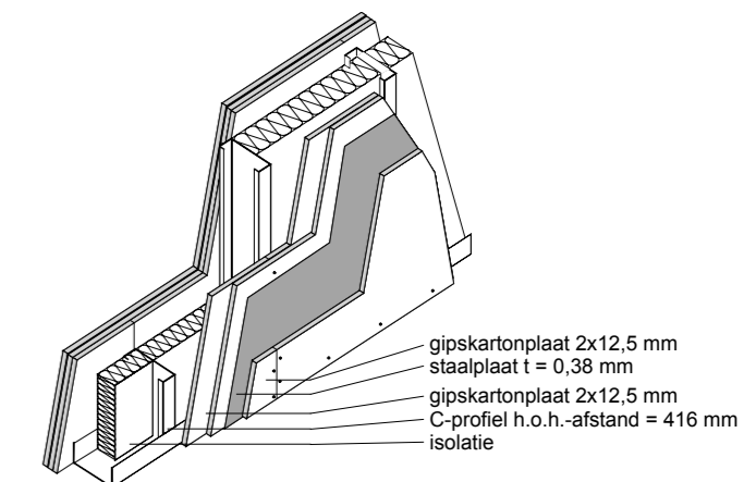
101. Brandwerendheid van een stabiliteitswand.
