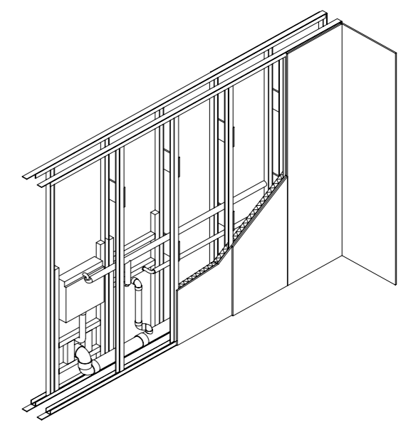
69. Dubbel uitgevoerde installatiewand. De stijlen zijn met plaatstroken aan elkaar verbonden.
