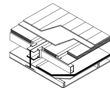
58. Vloeropbouw met een driedubbele ontkoppeling van de bekleding.
