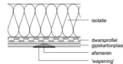
voegafdichting door 'gewapend' afsmeren
