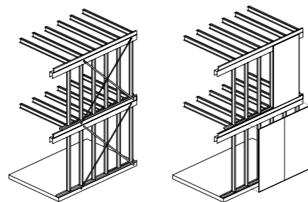
13. Stabiliteit met kruizen en schijfwerking uit beplating.
