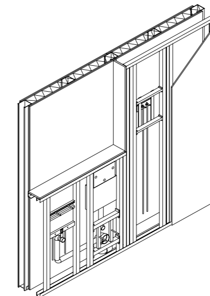
68. Voorzetwand voor inbouw van installaties (halfhoog en verdiepingshoog).
