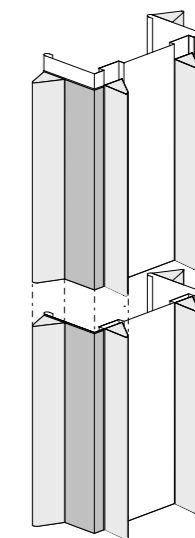
63. Metal-studprofiel met droge, rubberen geluidprofielen.
