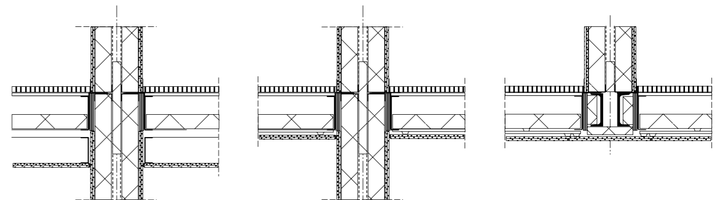
65. Detailoplossingen met I_{L_{LK}} > +5 dB.
