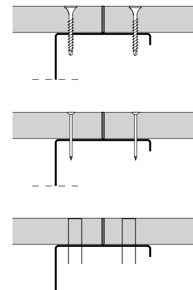
45. Verbindingsmogelijkheden van een beplating op staalframebouw.
