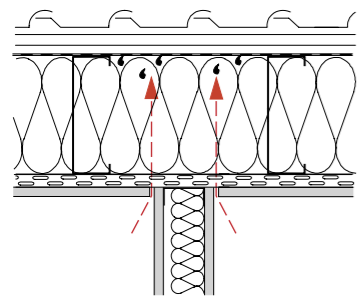
b open aansluiting bij een scheidingswand
