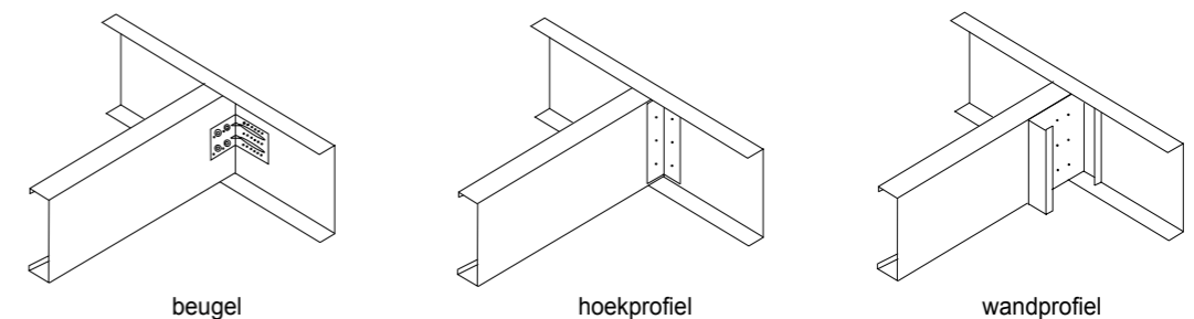
39. Plooiverstijvingen bij de opleggingen.
