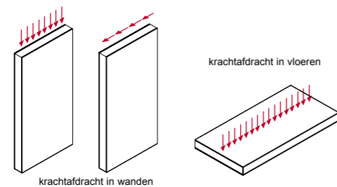
11. Schijfwerking uit horizontale en verticale elementen.
