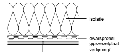
voegafdichting door verlijming of afsmeren
