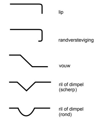
34. Verstevingen in het lijf of de flenzen.
