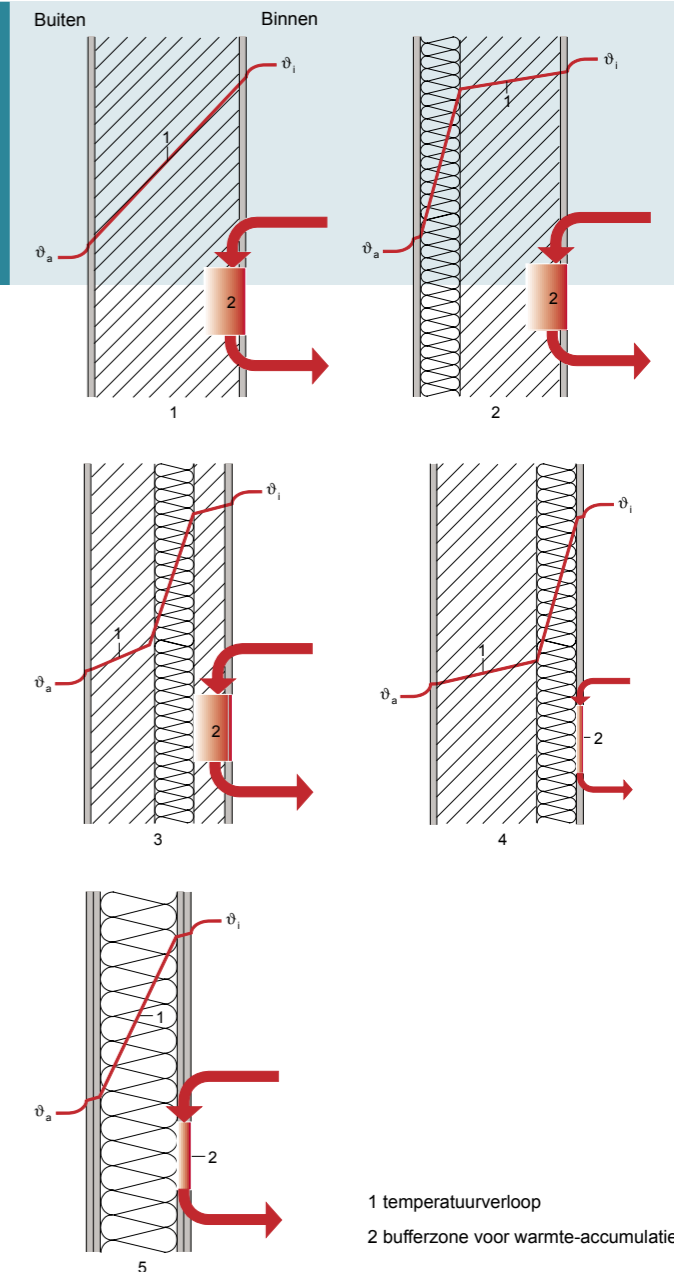
94. Warmte-accumulerend vermogen van verschillende wanden. 1 monoliet: het feitelijk warmte-accumulerend vermogen vindt slechts plaats over de eerste 80-100 mm. 2 wand met buitenisolatie. 3 een 'sandwich'-constructie: het warmte-accumulerend vermogen wordt bepaald door de dikte van het wanddeel aan de binnenzijde. 4 wand met binnenisolatie: binnenisolatie beperkt het warmte-accumulerend vermogen, maar verzorgt ook een snelle binnenverwarming. 5 inwendige isolatie: het warmte-accumulerend vermogen wordt bepaald door het materiaalgebruik van de binnenbekleding, isolatie en het staalframe (staaldikte en h.o.h.afstand).
