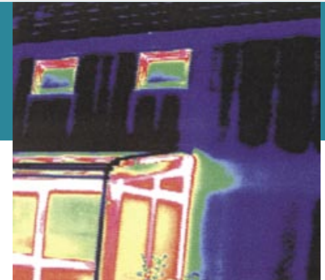
79. Thermovisuele weergave van een staalframebouw woning.
