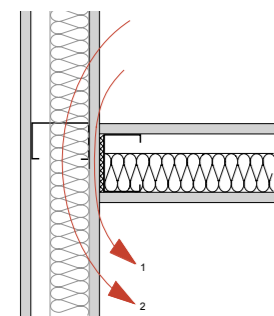
60. Geluidsoverdracht via het flankerende bouwdeel: 1. overdracht via de beplating; 2. overdracht via de holle ruimte (spouw).
