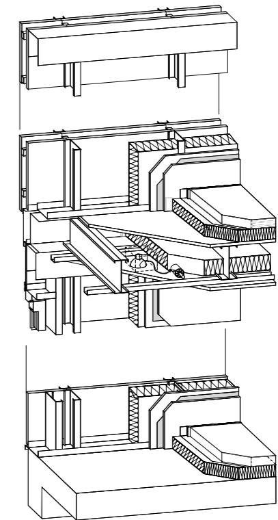
24. Ruwbouw en afbouw in staalframebouw.
