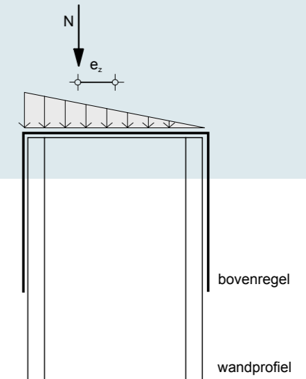
38. Excentrische belasting op een stijl.
