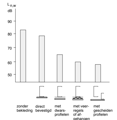
57. Vermindering van de geluidisolatie door het ontkoppelen van de onderbekleding van een vloer.
