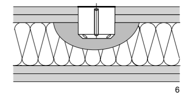
104. 'Protocol' voor het inbouwen van wandcontactdozen en wanden met een brandwerende functie.
