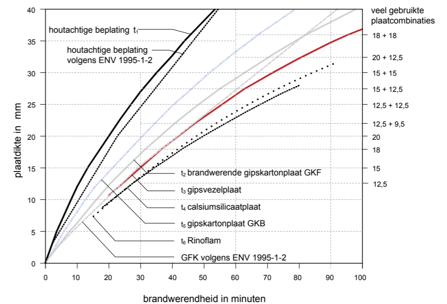
98. Karakteristieke doorbrandtijden van verschillende plaatmaterialen.
