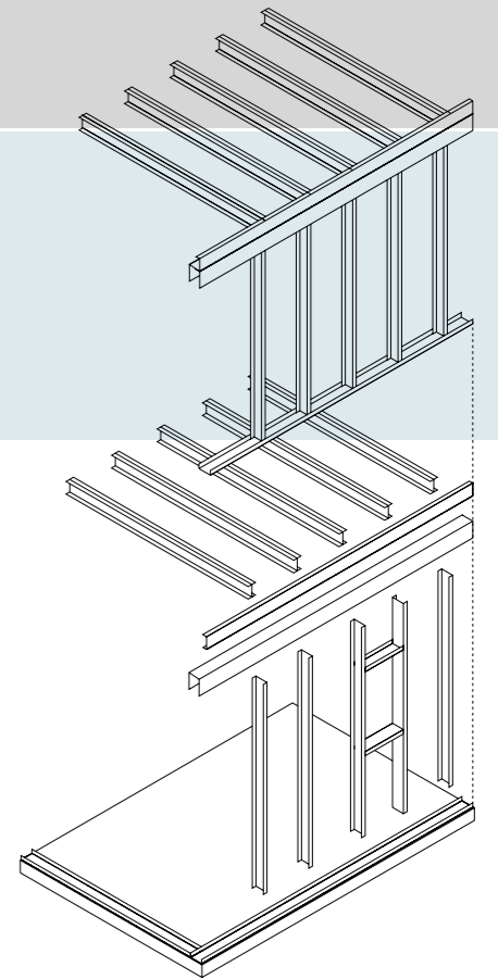
9. Constructieschema van staalframebouw.
