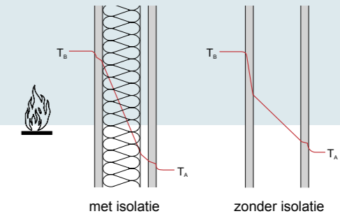
99. Temperatuurverloop in een scheidingswand met en zonder isolatie bij een eenzijdige brandhaard.
