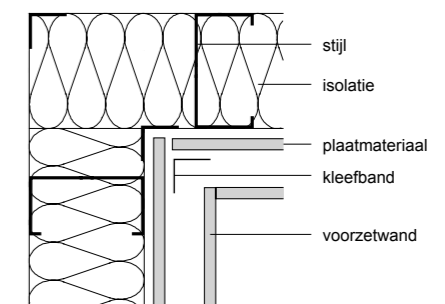
88. Luchtdichte uitvoeringen van een wandopbouw met plaatmateriaal.
