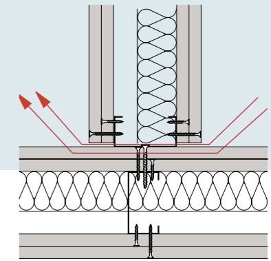
61. Akoestische 'lekken' en geluidbruggen bij een aansluiting van twee wanden.
