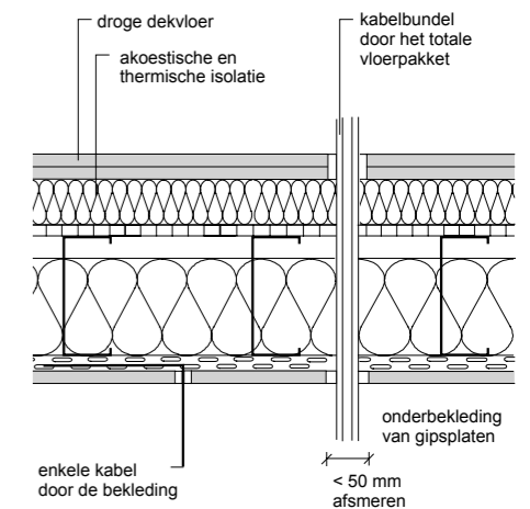
107. Brandwerende uitvoering van openingen en doorvoeren in staalframebouw vloeren.
