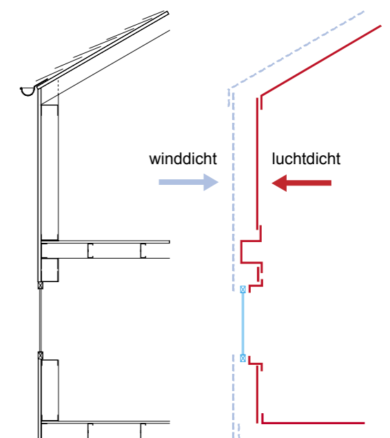
86. Verschil tussen winddicht en luchtdicht.
